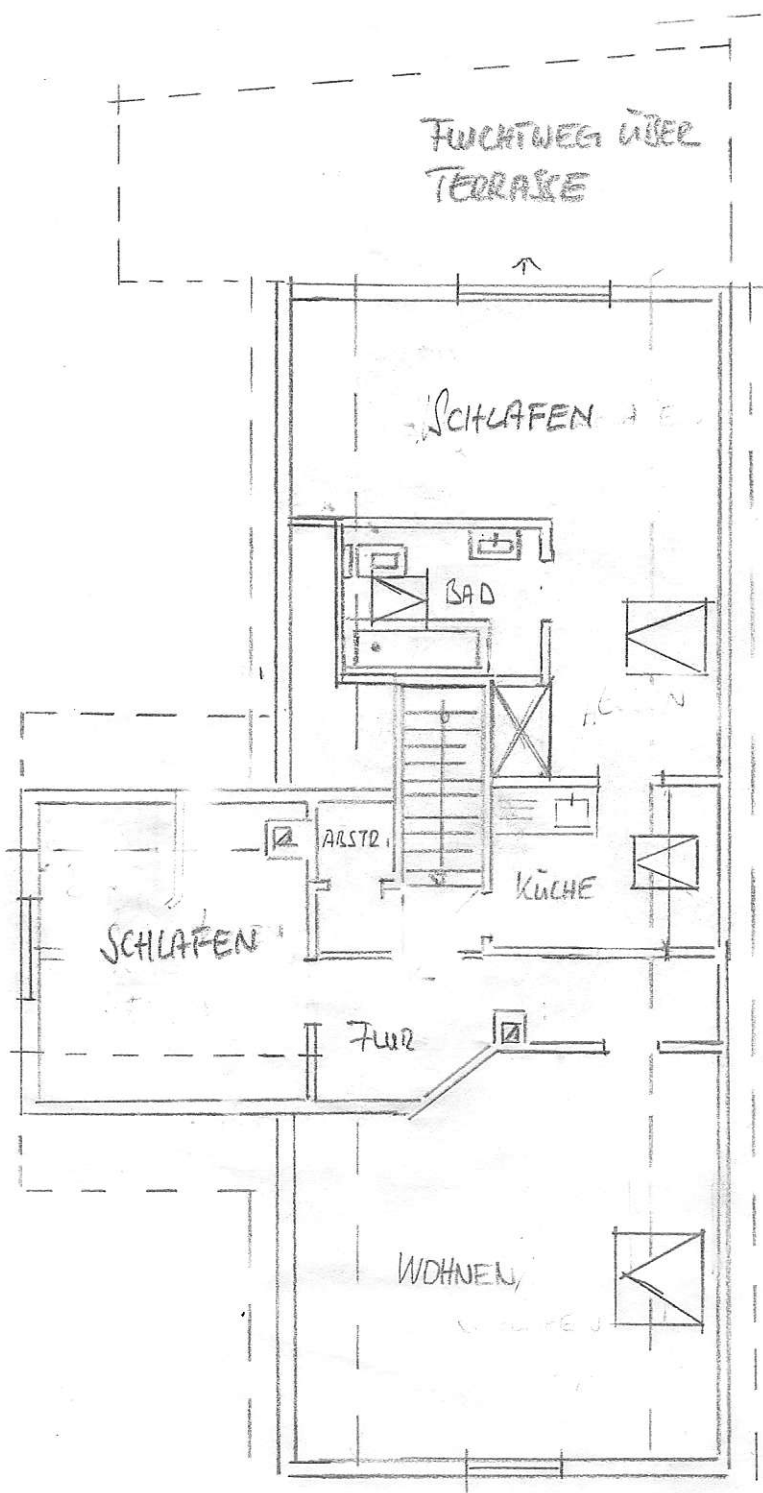
DACHGESCHOSS 1 WE M 1:100
